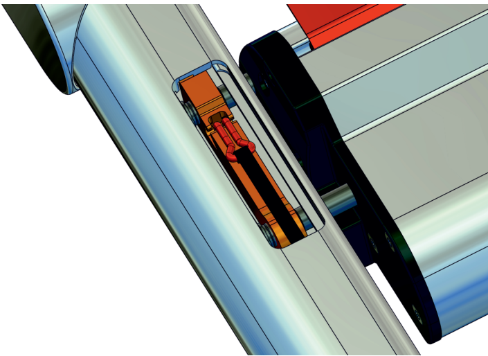
Zughaken „links“ eingehängt!
