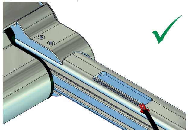
Zughaken „rechts“ vormontiert
